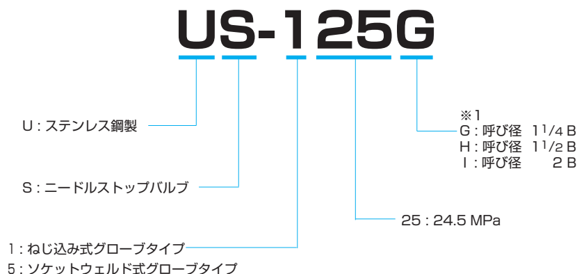
※1: ねじのサイズ (管用テーバねじの場合)
